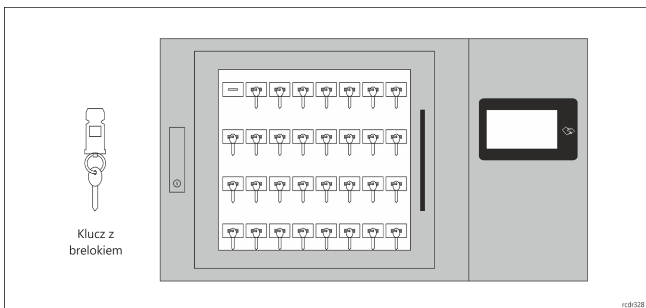
Rys. 1 Widok ogólny depozytora RKD32
